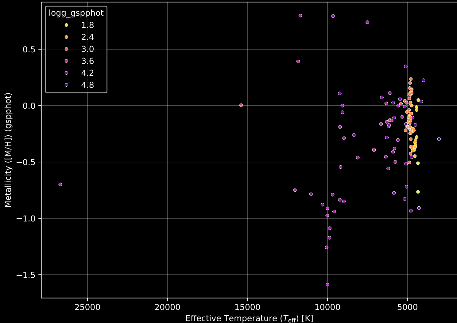
APOGEE DR17 Field: [N6819-RV_btx] Stellar Population Parameters (n= 137)
